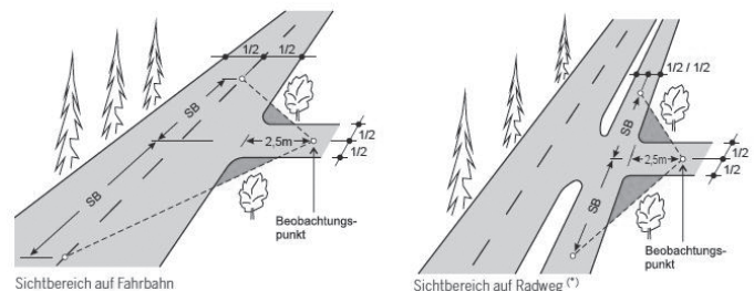
C: Minimal freizuhaltende Sichtbereiche Knotenbereich (Einführungen und Kreuzungen)
