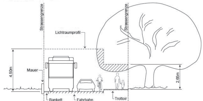
B: Minimale seitliche Abstände
